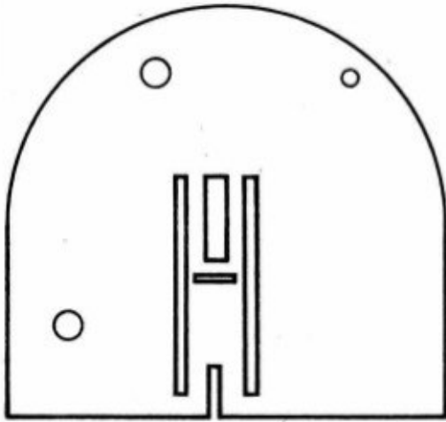
8004 0902 Stichplatte für ZZ-Stich 8014/25, /25-2, /35, /35-2, /29, /43 und 8014/40 mit Graugussgrundplatte
