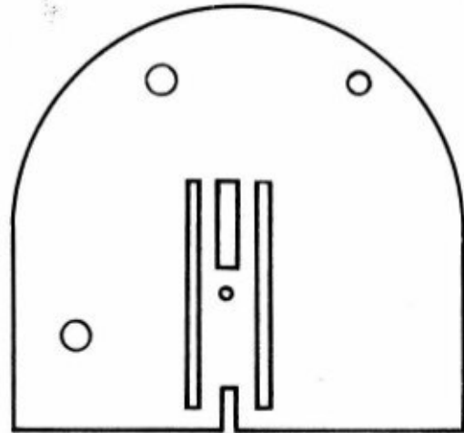
8004 1306 Stichplatte für Geradstich der Klassen 8014/26, 8014/261 und 8014/36
