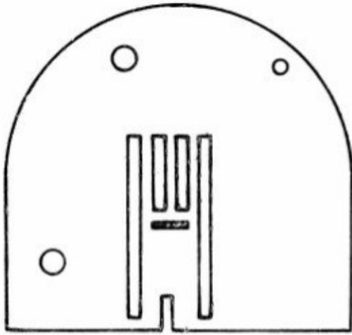
8002 2042 Stichplatte für ZZ-Stich Baureihe Rubina mit Grauguss-Grundplatte
