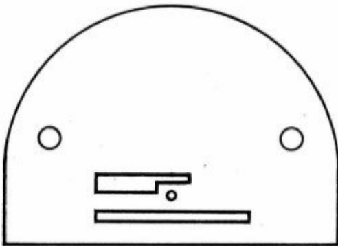
8008 1762 (121711) Stichplatte für ZZ-Stich der Klassen 8014/2-3 und 8014/22-33
