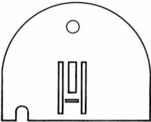
8002 0102 Stichplatte für ZZ-Stichplatte der Klassen 8014/26 und 8014/36
