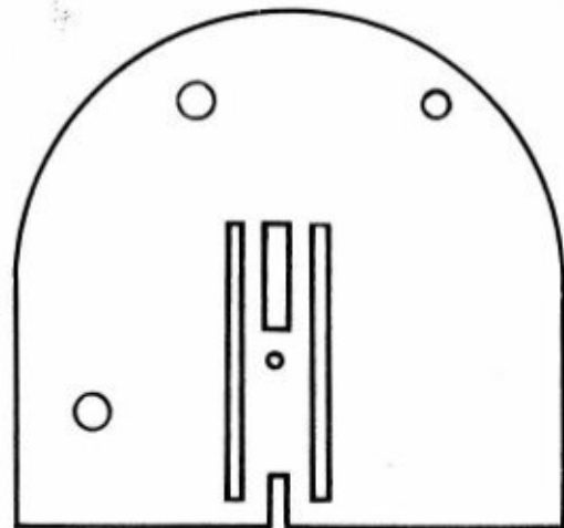
8004 1306 Stichplatte für Geradstich 8014/25, /25-2, /35, /35-2, /29, /43 und 8014/40 mit Graugussgrundplatte
