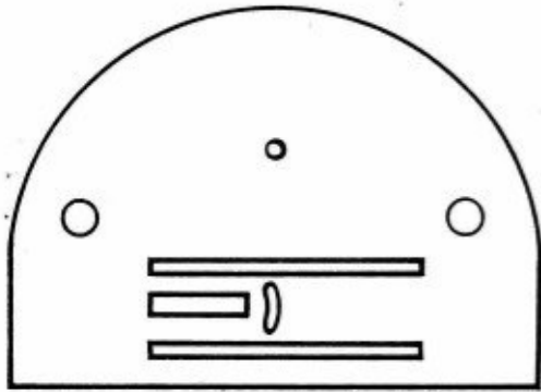
8008 1762 (121711) Stichplatte für ZZ-Stich der Klassen 8014/2-3 und 8014/22-33
