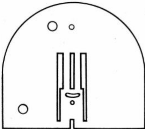
8008 1881 (8010-2.10) bzw. (141709) Stichplatte für Klasse 8010 und 8014/4
