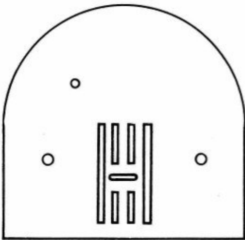
90-02-038 Stichplatte für Geradstich der Klasse 466 Import VR Polen
