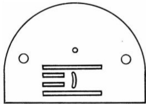
430-04-261 Stichplatte für ZZ-Stich der Klasse 466 Import VR Polen
