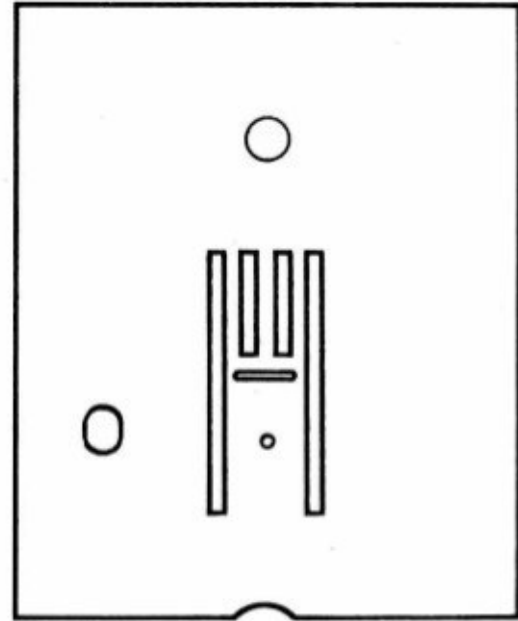
8002 0719 Stichplatte für Geradstich der Klasse 8014/44
